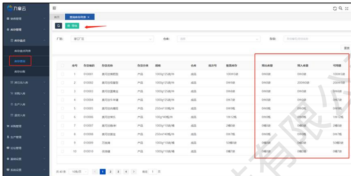
图 4-2-1 库存查询
