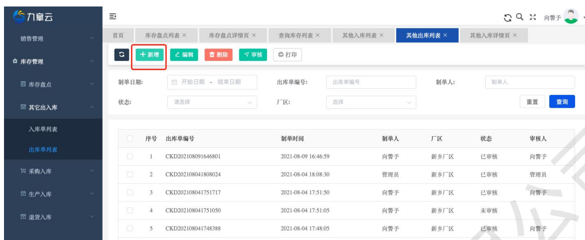
图 4-4-2-1 出库单列表
