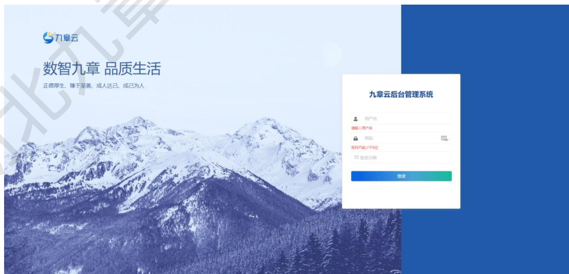
图 3-1 登录页面
